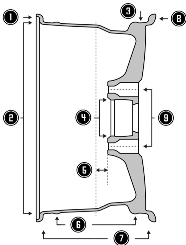
1: Fælghorn (inderste), 2: Diameter, 3: Skulder, 4: Centerhul, 5: Indpresning, 6: Hump, 7: Bredde, 8: Fælghorn (ydre), 9: Hulafstand
